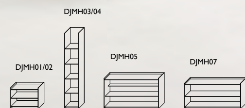
DJMH01 L30 - P45 - H45,5 DJMH02 L60 - P45 - H45,5 DJMH03 L30 - P45 - H195,5 DJMH04 L60 - P45 - H195,5 DJMH05 L120 - P45 - H107,5 DJMH07 L120 - P45 - H54,5
